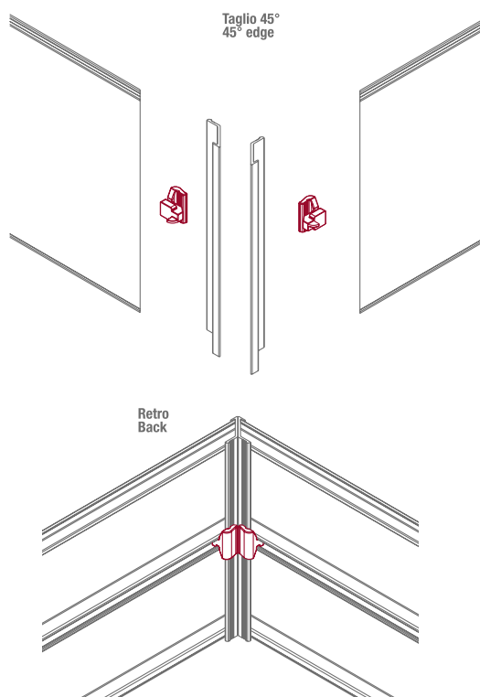
Clip di fissaggio per zoccolo in plastica per art. 1359 e 1360 For plastic plinth fixing clip for 1359 and 1360 ART. CSP02391-07SF
