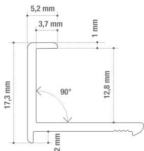
Angolare 90° in alluminio – Taglio 90° 90° aluminium corner bracket – 90° Edge ART. 1359
