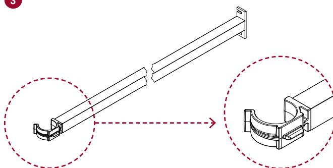
Coppia di clip per fissaggio piedino predisposta per gancio GZ58 Pair of fixing clips for leg compatible with GZ58 clip-type connector CSP0337
